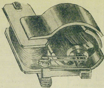
Общий вид мотора (сильно увеличено).
