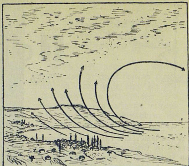
Так в жаркий день на берегу моря рождается бриз.
