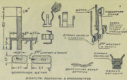
Чертеж 1. Детали индуктора.
