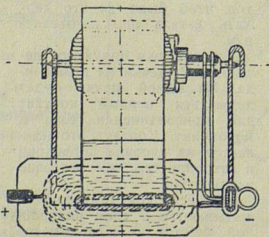
Чертеж 2 и 3. Изготовление якоря и коллектора.
