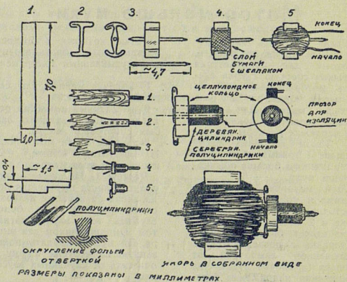
Чертеж 2 и 3. Изготовление якоря и коллектора.
